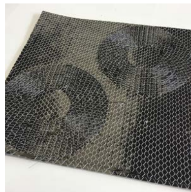
円形繊維プリフォーム
