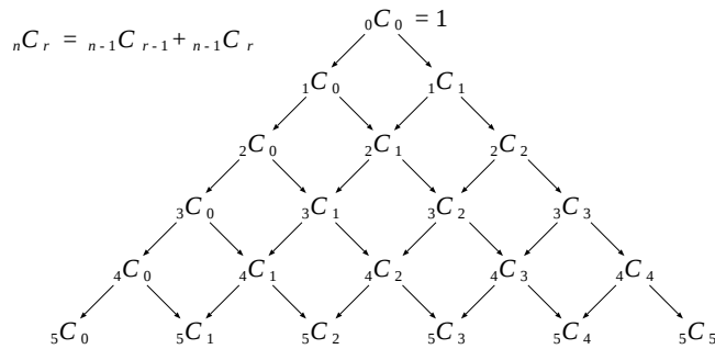
図 1: Pascal の三角形による nC_r の計算。漸化式 nC_r = {}_{n-1}C_{r-1} + {}_{n-1}C_r が成立するので、矢印の根本の数字を足し合わせることで矢印の先の数を計算できる。 {}_0C_0 = 1 から始めて、順に {}_1C_0, {}_1C_1, {}_2C_0, {}_2C_1, {}_2C_2, \dots を求めることで、全ての nC_r が得られる。
