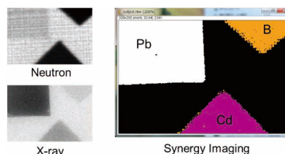
Fig.3 Element distribution map by neutron and X-ray synergy imaging. 図3 中性子/X線相乗イメージングによる元素分布マップ。
