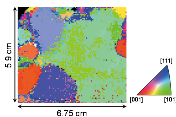
Fig.2 Crystal grain map with their orientations by neutron Bragg-dip transmission method. 図2 中性子ブラッグディップ透過法による結晶粒と方位のマップ。
