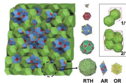
図2 Yb-Cd正20面体準結晶の構造モデル(RTH、AR、ORはクラスター構造単位を示し、黒枠内に対応する近似結晶でのクラスター配列を示した)
