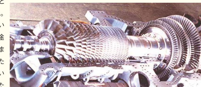
▲発電用ガスタービン 材料には部位ごとに異なる特性が要求され材料技術者にとって挑戦の場。
