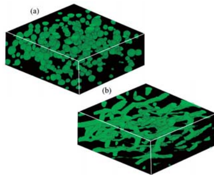
図2 電場をかけたときの粘度の低いドロップレット構造(a)から粘度の高いネットワーク構造(b)への変化
