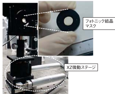
図1 開発中の観測装置の心臓部となるフォトニック結晶マスク
