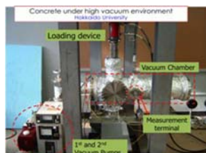
図3 高真空環境下における載荷試験装置
