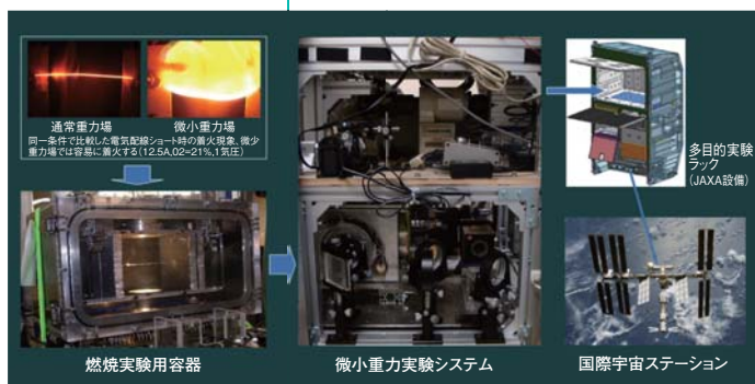
図1 ISS火災安全性実験に向けた装置開発
